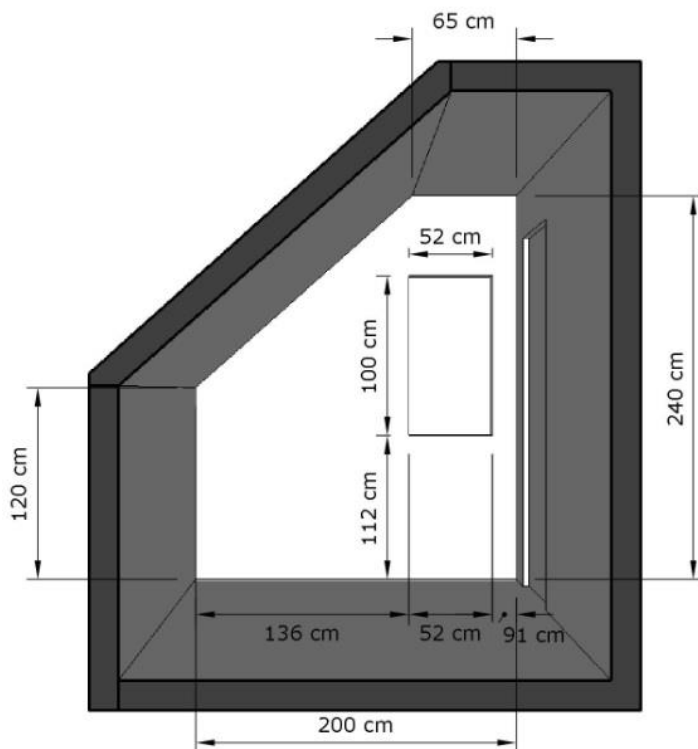
Rys. 2 - Widok od boku
